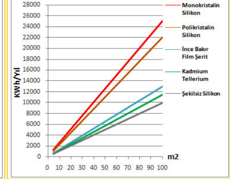
TÜRKİYE PV Tipi Alan Üretililecek Enerji (KWh-Yıl)
